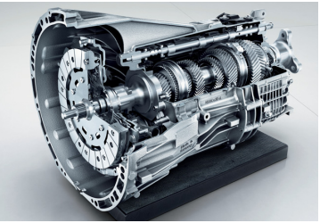
6速マニュアルトランスミッション
